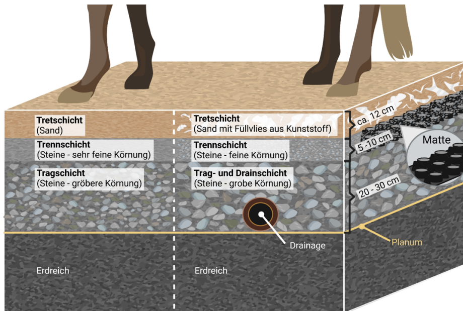
Abbildung 1: Beispielhafter Aufbau eines Reitplatzes. Dargestellt sind zwei Optionen. Der Aufbau auf der linken Seite beinhaltet in der Tretschicht nur Reitsand. Dieser Aufbau ist aufgrund der nicht immer optimalen Eigenschaften sehr viel seltener als der rechts dargestellte Aufbau mit Zuschlagstoffen. Erstellt mit (BioRender.com, 2022). Entnommen aus [1].
